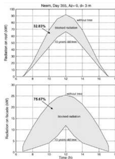
Sombreamento de uma árvore no telhado de um edifício (em cima) e na parede sul (em baixo) (Gómez-Muñoz et al., 2010)
